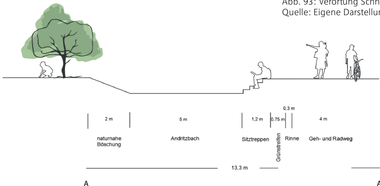
Abb. 94: Schnitt A am Andritz Bach beim Strasserhofweg, Quelle: Eigene Darstellung
