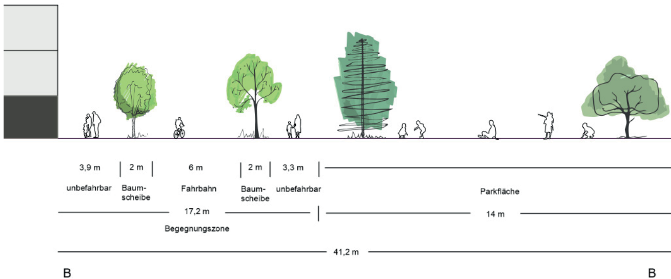
Abb. 108: Schnitt B Zentrum an der Grazer Straße, Quelle: Eigene Darstellung
